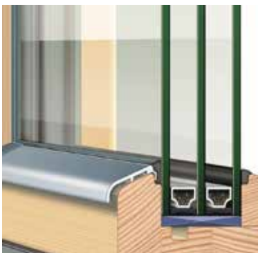
3-Scheiben Wärmeschutzverglasung
