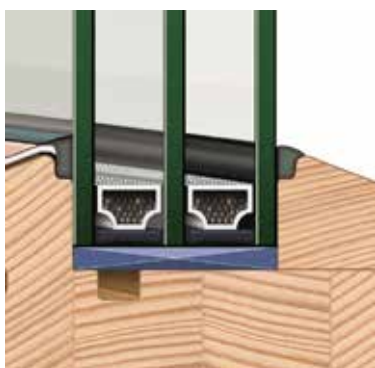
3-Scheiben Wärmeschutzverglasung
